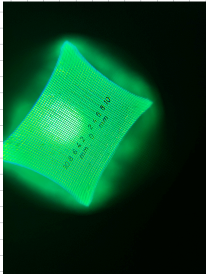
Abbildung 3.7: Kreuzgitter
